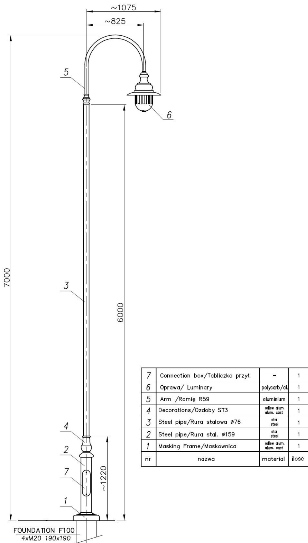
Przykładowy wizerunek elementu słupa
