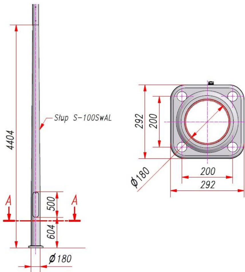
Przykładowy wizerunek elementu słupa
