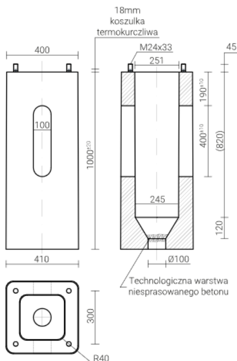
Przykładowy wizerunek fundamentu prefabrykowanego
