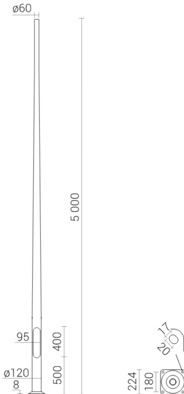
Przykładowy wizerunek elementu słupa
