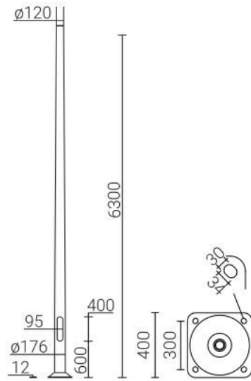
Przykładowy wizerunek elementu słupa
