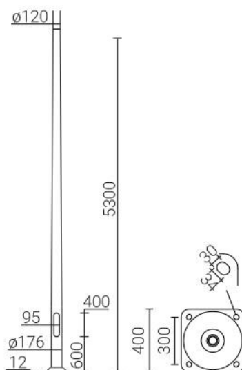
Przykładowy wizerunek elementu słupa
