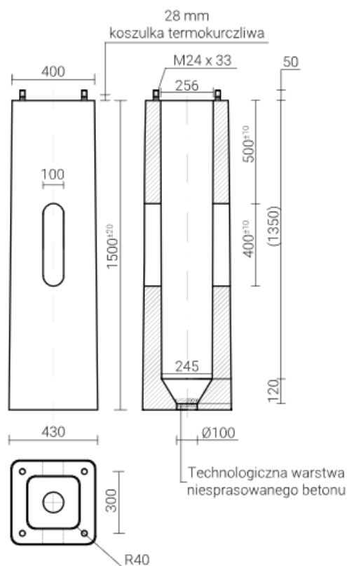
Przykładowy wizerunek fundamentu prefabrykowanego
