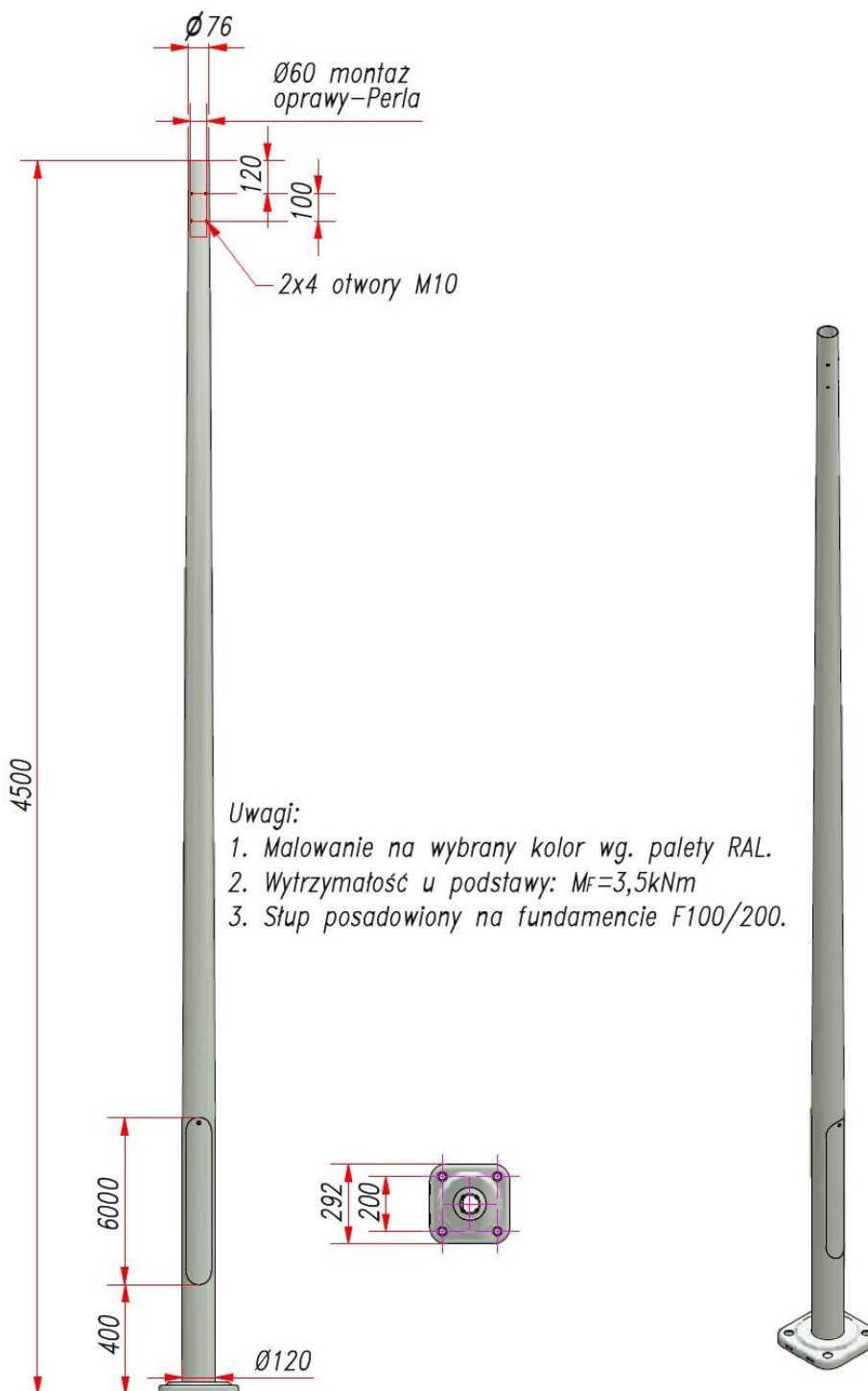
Przykładowy wizerunek elementu słupa
