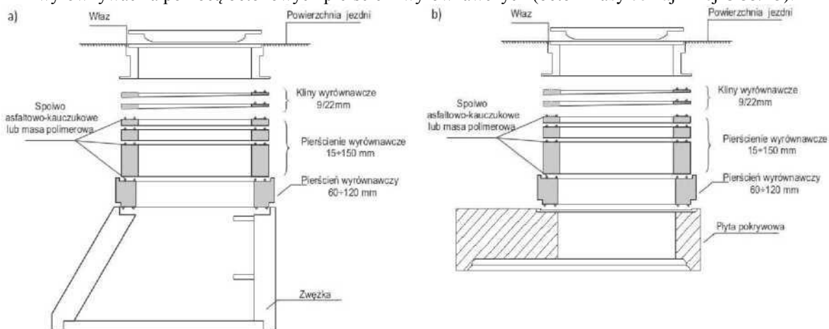
Rys. 1. Schemat przykładowego montażu pierścieni wyrównawczych dla dwóch przypadków a) z elementem przejściowym (zweżką), b) z płytą nastudzienną
